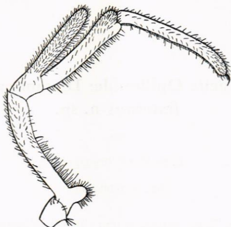
Abb. 1 Dicranopalpus fraternus n. sp. Linke Pedipalpe innenseits.
